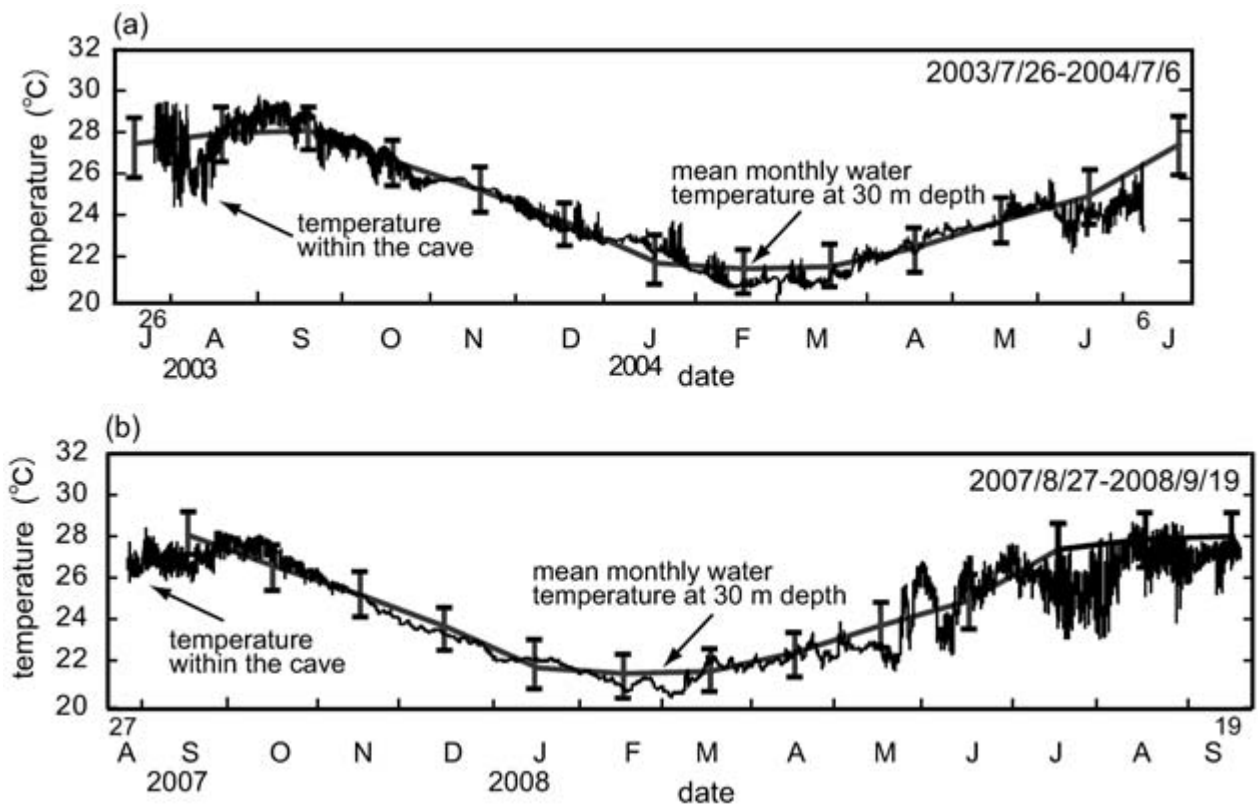
図2 海底洞窟“大洞窟”内の水温と沖縄海域（北緯26－27°，東経127－128°）の水深30mの月平均水温との比較。(a) 2003年7月26日から2004年7月6日までの期間 (Kitamura et al. , 2007). (b) 2007年8月27日から2008年9月19日までの海底洞窟“大洞窟”内の水温。月平均水温のデータは日本海洋センター ( http://jdoss1.jodc.go.jp/cgi-bin/1997/bts.jp ) に基づく。
